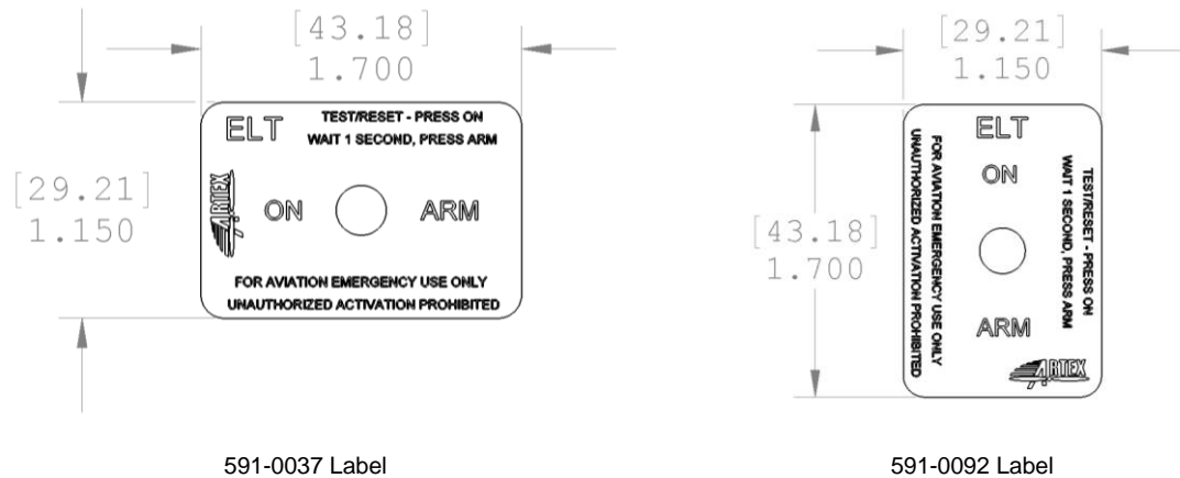
Figure 6 : Label 591-0037 & 591-0092
